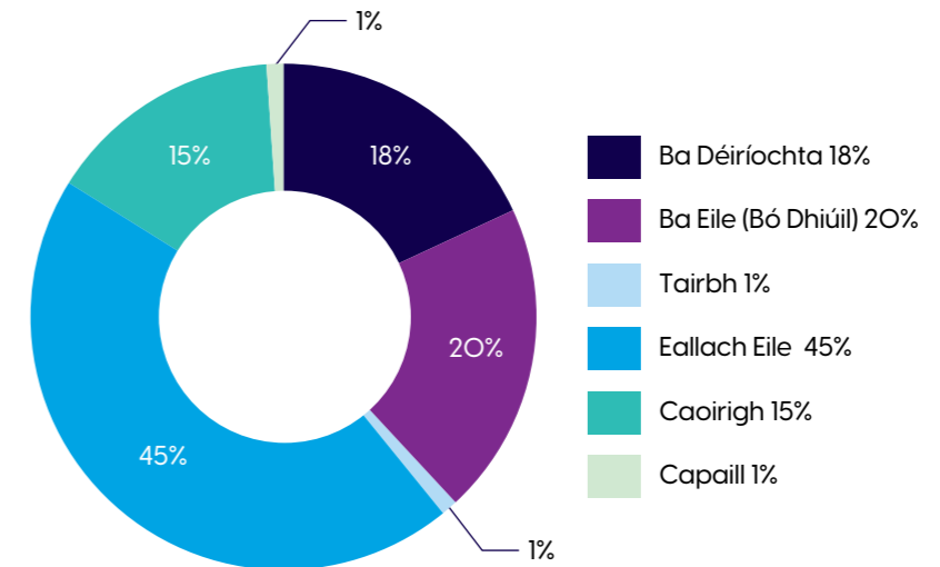
Figiúr 3-12: Astaíochtaí Talmhaíochta Chill Dara
