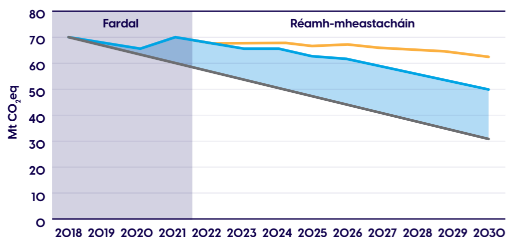
Figiúr 2-6: Iomlán astaíochtaí GCT na hÉireann le bearta aeráide reatha (oráiste) agus bearta breise aeráide (gorm) go dtí 2030 i gcomparáid leis an sprioc laghdaithe de 51% (liath) (GCC, 2023)
