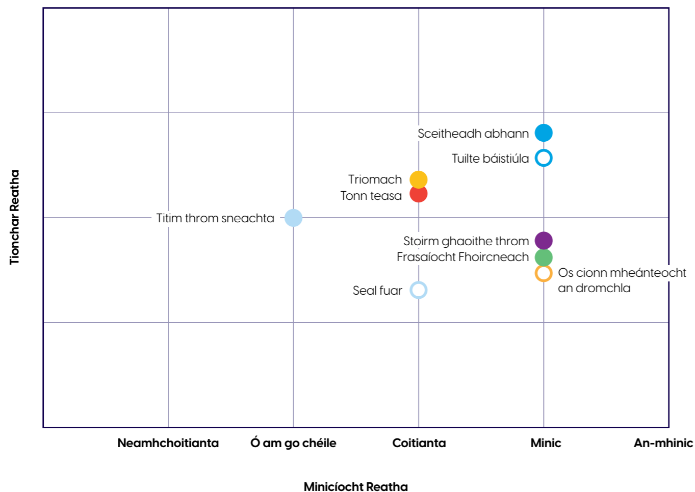
Figiúr 3-3: Maitrís Tionchair Aeráide Reatha
