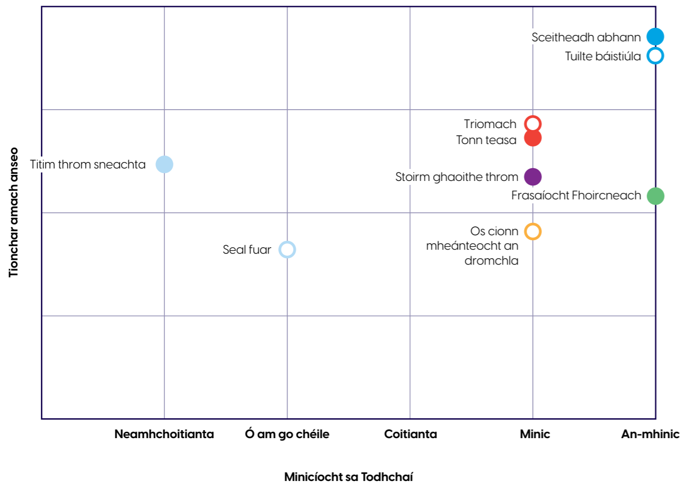
Figiúr 3-4: Maitris Tionchair Aeráide Amach Anseo
