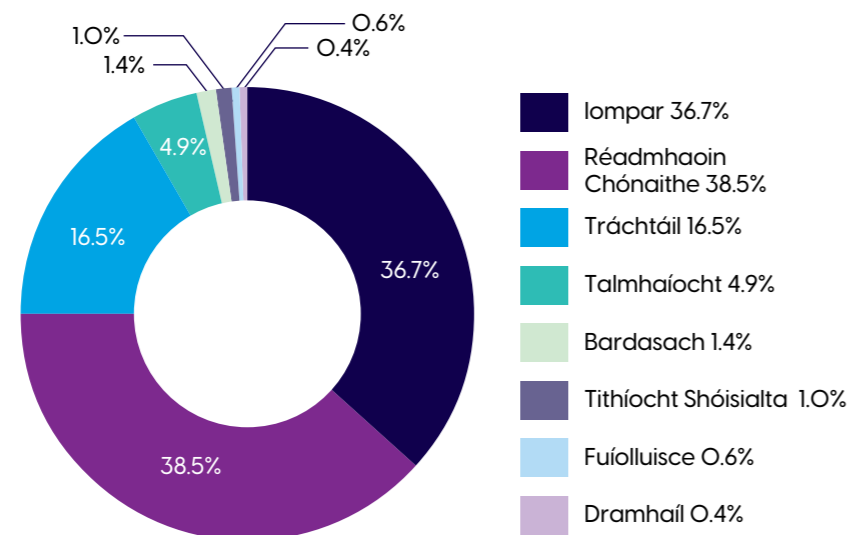
Figíur 5-2: Bonnline Earnála agus Iomlán 2018 do CD Mhaigh Nuad
