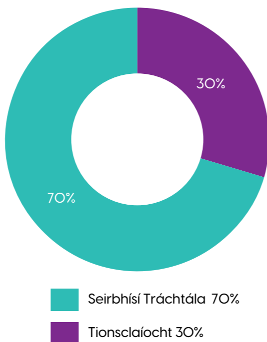
Figiúr 3-8: Astaíochtaí na hEarnála Bardasaí (tCO 2 e)
