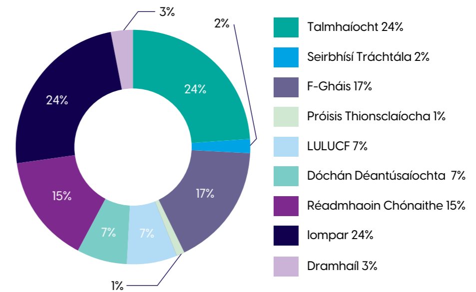
Miondealú Earnálach CO 2e MapÉire
