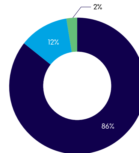
Figiúr 3-9: Astaíochtaí na hEarnála Bardasaí (tCO 2 e)
