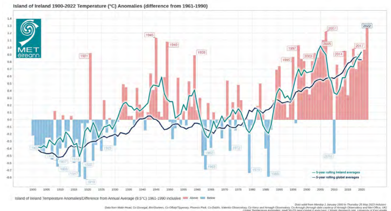
Figiúr 2-2: Aimhrialtachtaí Teochta (°C) Oileán na hÉireann 1900-2022 (dífeár ó 1961-1990) (Foinsé: Met Éireann)
