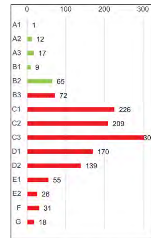
Figiúr 3-10: Stoc Tithíochta Sóisialta RFFanna (Uimh)
