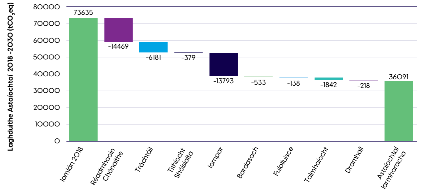
Figíur 5-3: Scála Laghdaithe Astaíochtaí Earnála do CD Mhaigh Nuad
