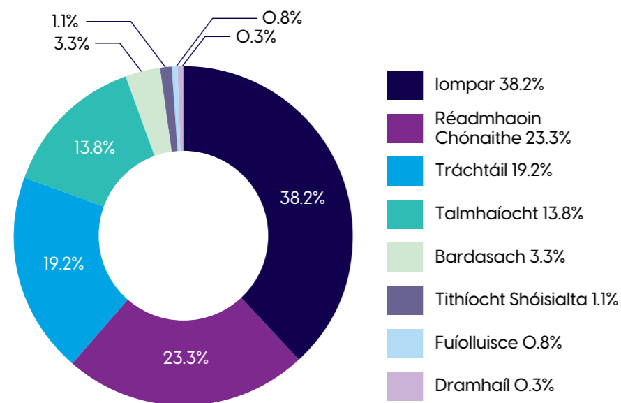
Figiúr 3-5: Próifil Astaíochtaí 2018 do Chontae Chill Dara
