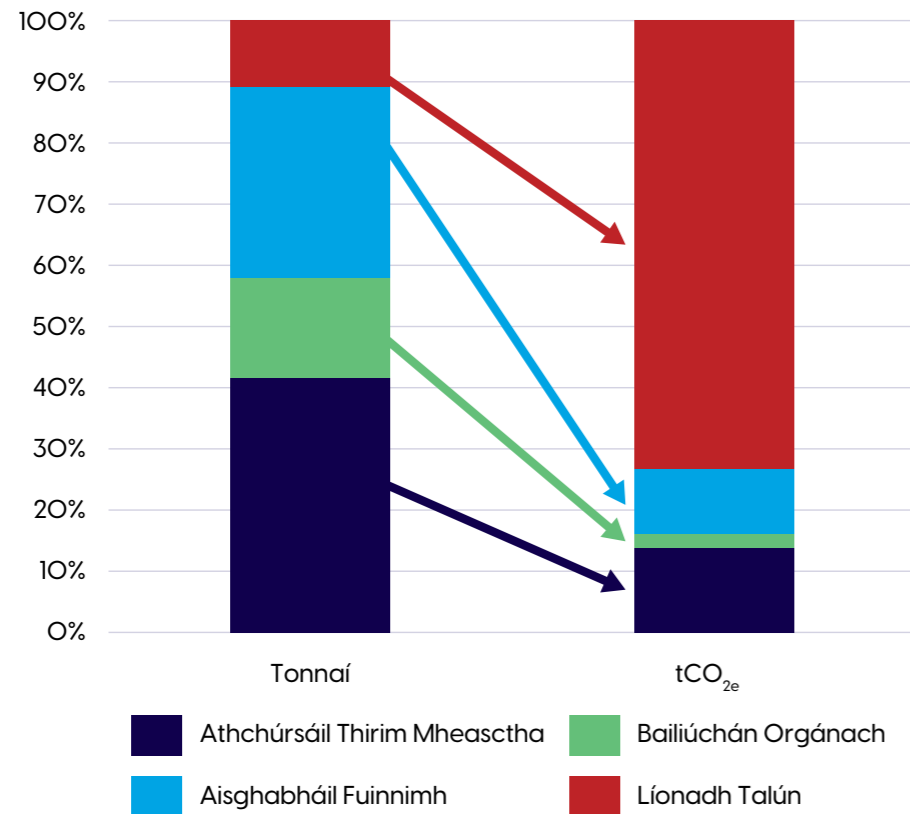
Figiúr 3-11: Astaíochtaí Earnáil Dramhaíola Chill Dara
