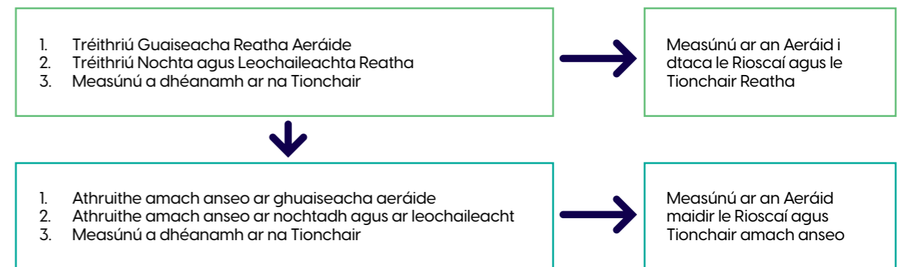
Figiúr 3-1: Modheolaíocht Measúnaithe Riosca um Athrú Aeráide
